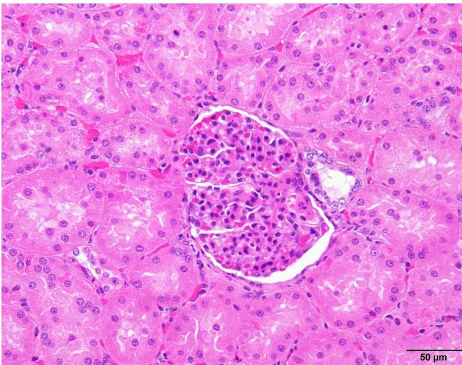
2倍カラッツィヘマトキシリン（検体：豚の腎臓）
