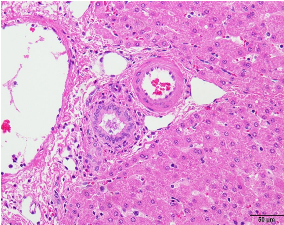
2倍カラッツィヘマトキシリン（検体：豚の肝臓）
